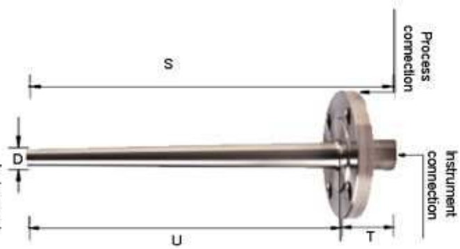
BAR STOCK FLANGE THERMOWELL
